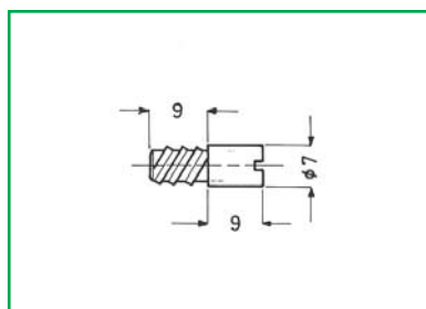
Perno filetto mordente Bolt with raised thread Gewindebolzen zum direkten Einschrauben Tige avec filet auto-filetant Perno rosca madera
